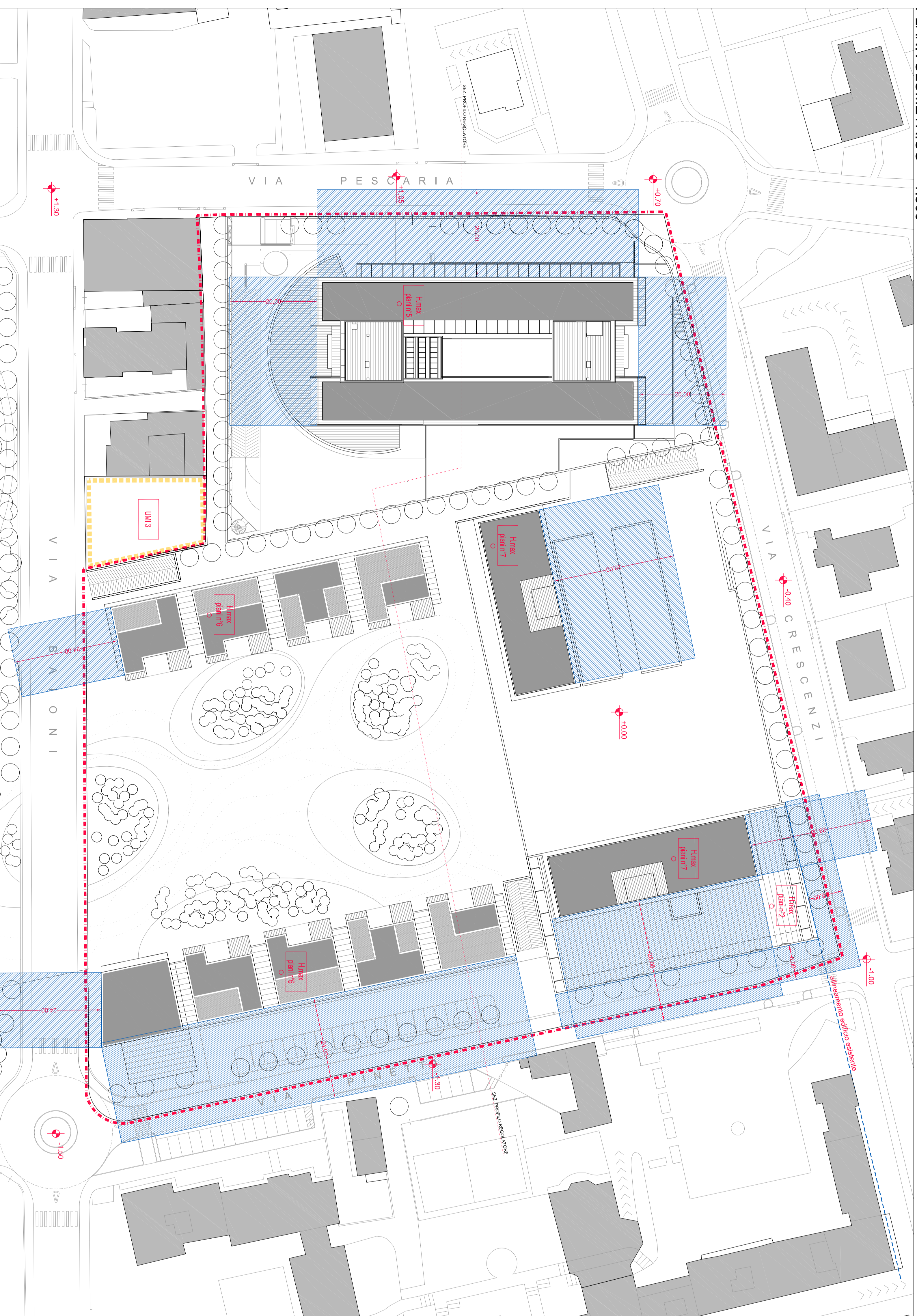
PLANIVOLUMETRICO 1:500
